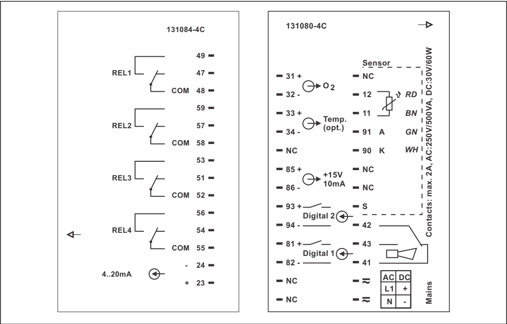
11 盘装型变送器的接线腔粘贴标签示意图
