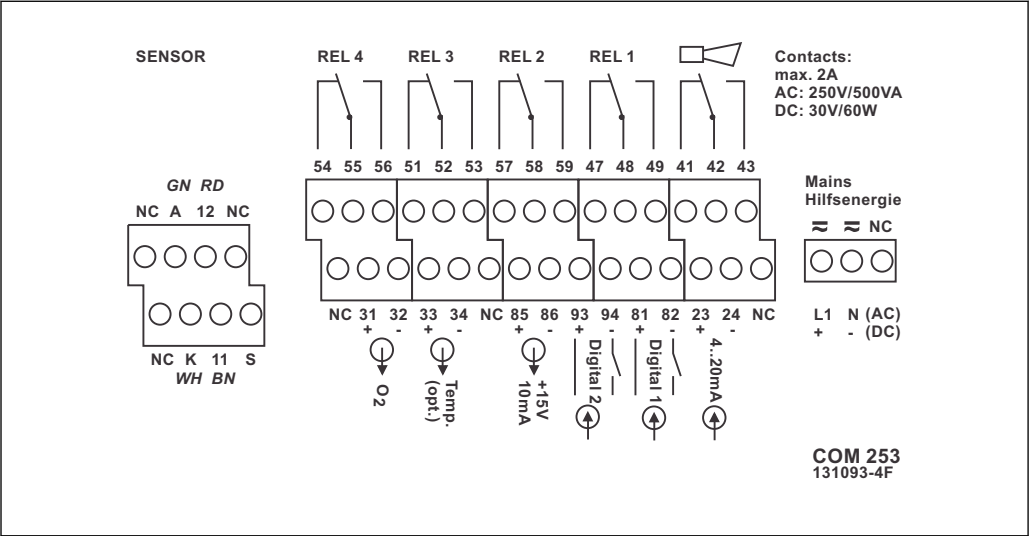
10 现场型变送器接线腔内的粘贴标签示意图
