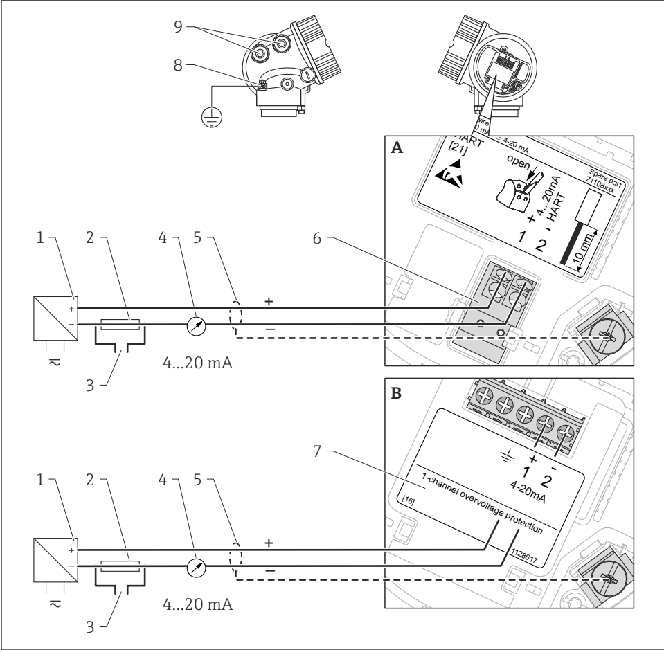
图 8 两线制连接的接线端子分配示意图; 4...20 mA HART
