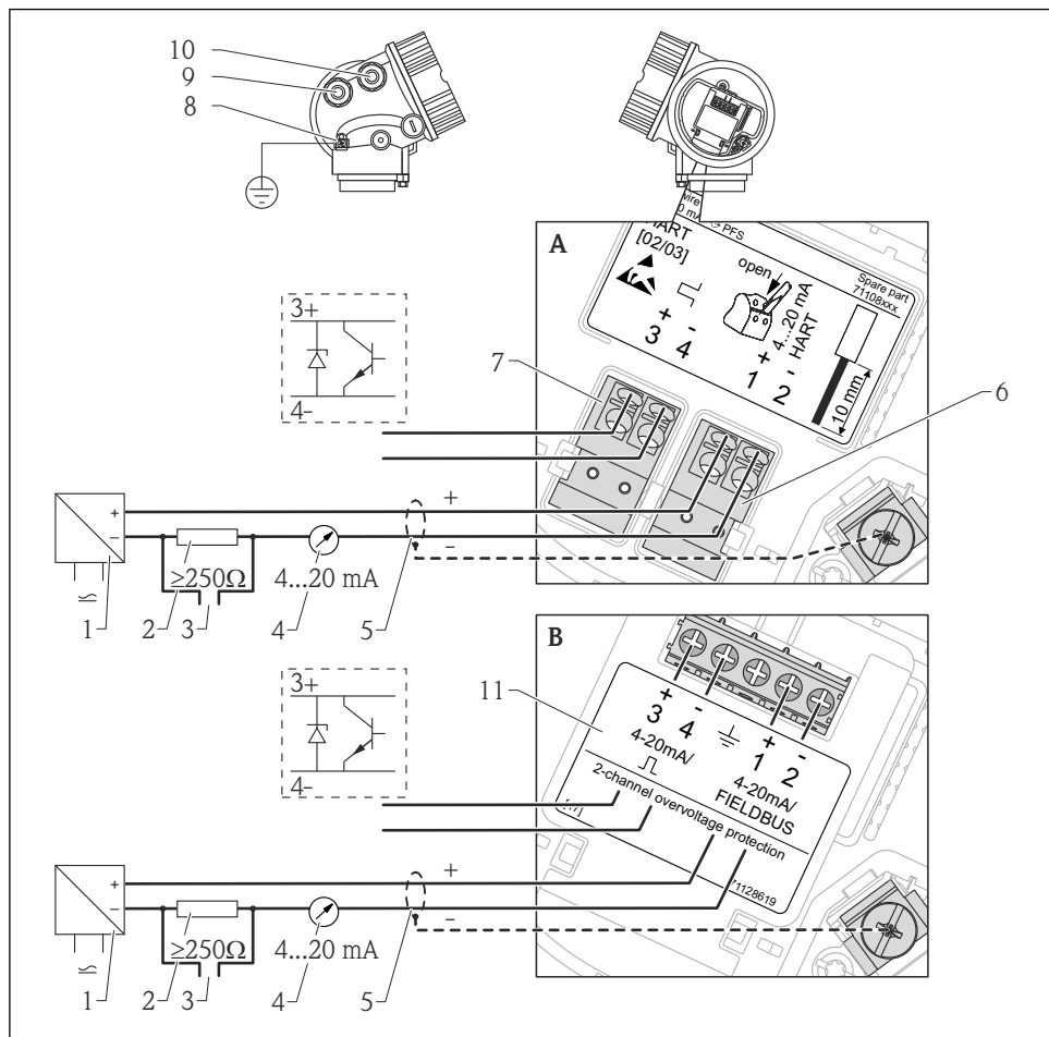
图 9 两线制连接的接线端子分配示意图; 4...20 mA HART, 开关量输出
