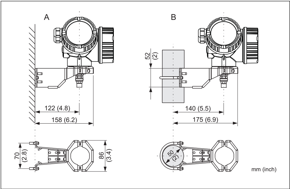
图 6 使用安装支架安装电子腔外壳
