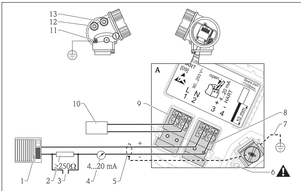
12 四线制连接的接线端子分配示意图; 4...20 mA HART (90...253 V AC)
