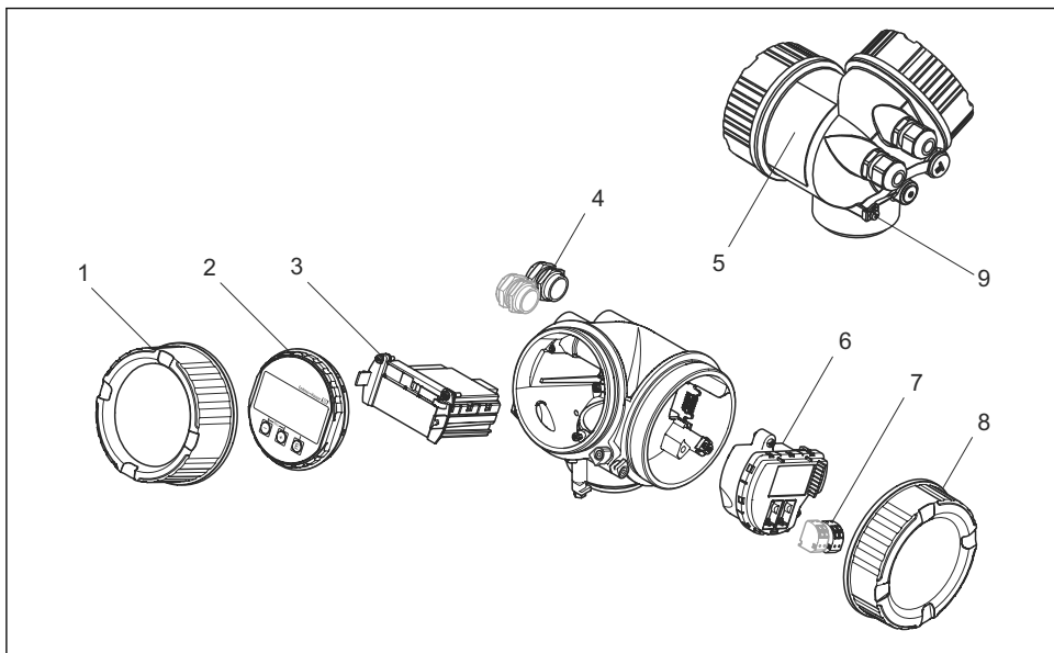
图 2 电子腔外壳的结构示意图
