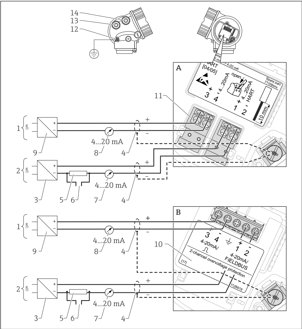
10 两线制连接的接线端子分配示意图; 4...20 mA HART, 4...20 mA
