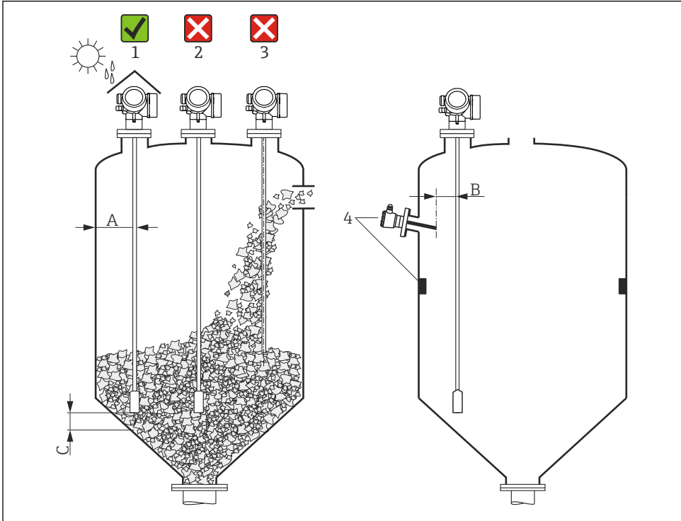
图 4 Levelflex 的安装位置
