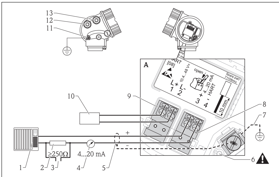
11 四线制连接的接线端子分配示意图; 4...20 mA HART (10.4...48 V DC)
