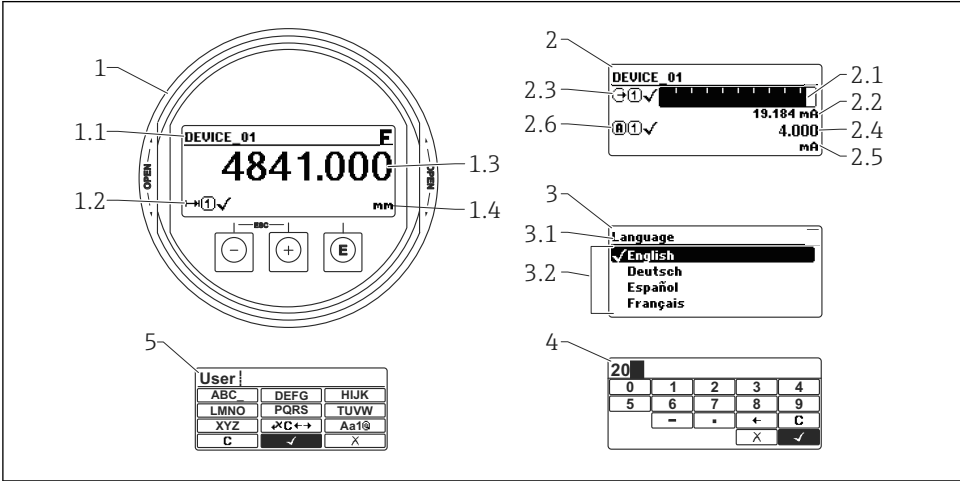
15 现场操作的显示与操作单元示意图
